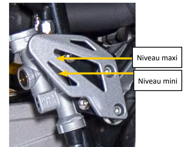
Maître-cylindre arrière
