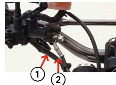
1. Contre-écrou 2. Ecrou de réglage
